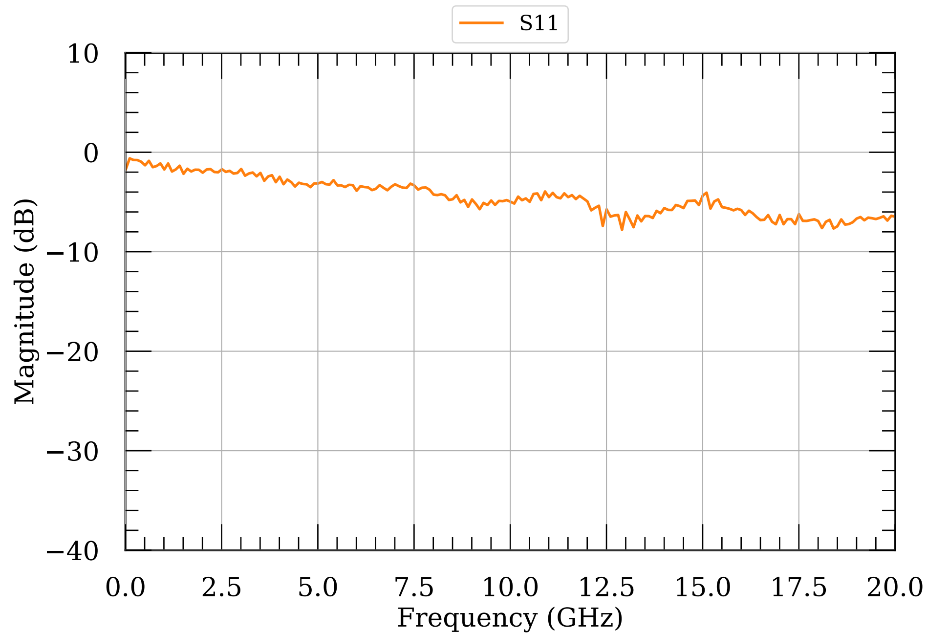
LNA S-params module045
